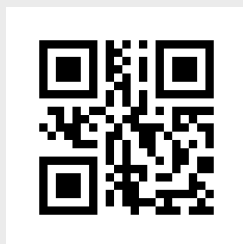
回车换行
