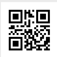
* 启用补光灯
