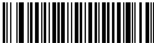
* 8 BPP
