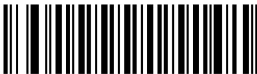
Aktivieren MSI
