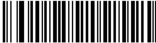
TIFF-Dateiformat
