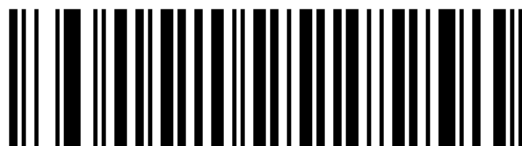
* CLSI-Bearbeitung deaktivieren
