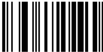
Eingabe abbrechen
