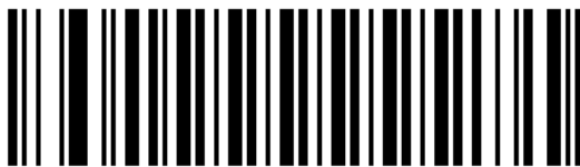
禁用 Code 39
